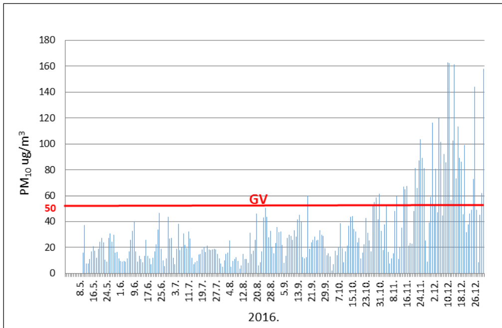
Slika 3.3. Kretanje srednjih 24-satnih koncentracija PM 10 tijekom 2016. (Izrađeno prema podacima Ekonerga, 2017.)
