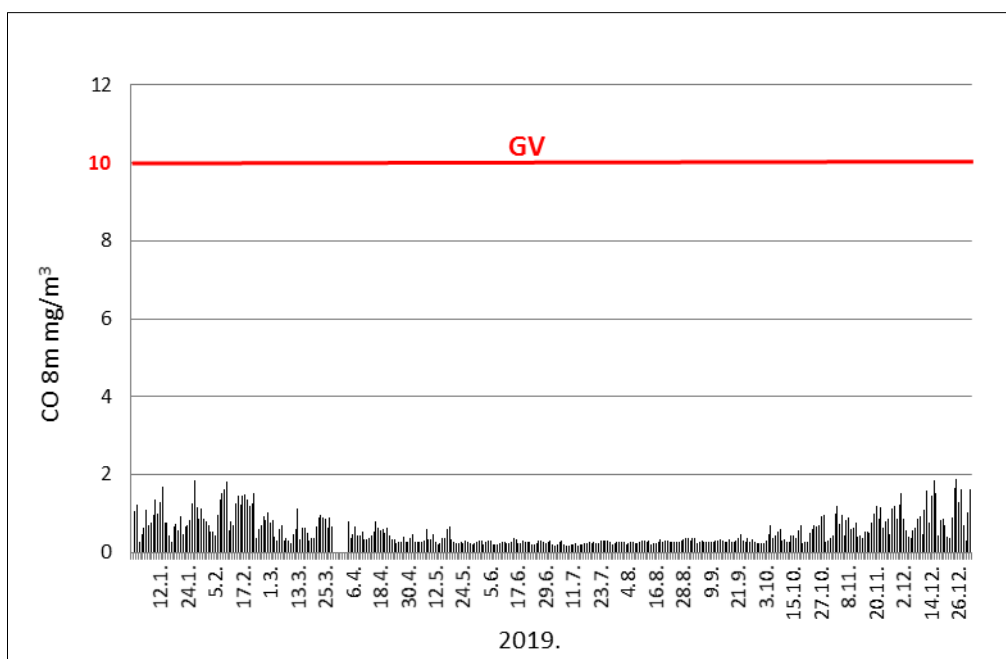
Slika 3.10. Kretanje srednjih 8-satnih koncentracija CO tijekom 2019. (Izrađeno prema podacima Ekonerga, 2020.)
