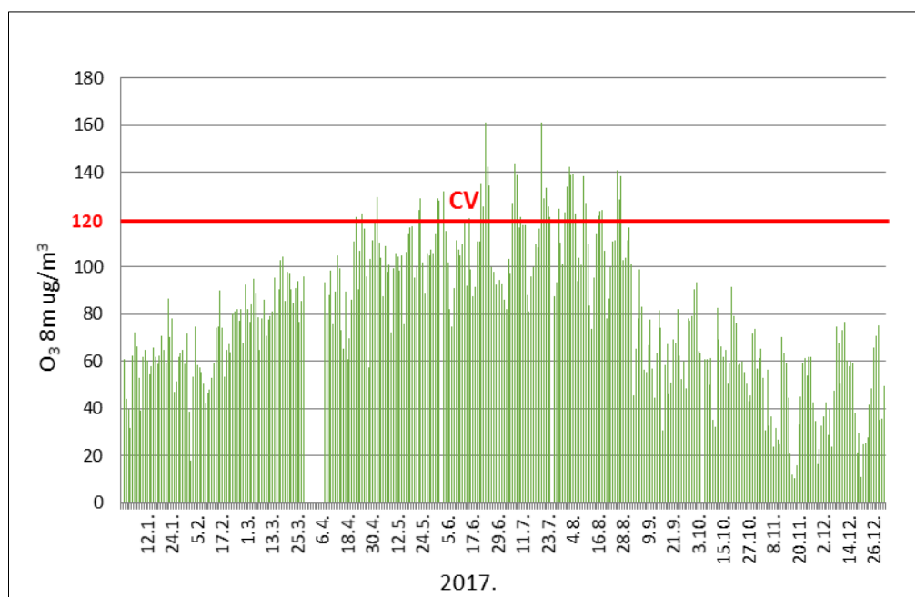
Slika 3.12. Kretanje srednjih 8-satnih koncentracija O_3 tijekom 2017. (Izrađeno prema podacima Ekonerga, 2018.)
