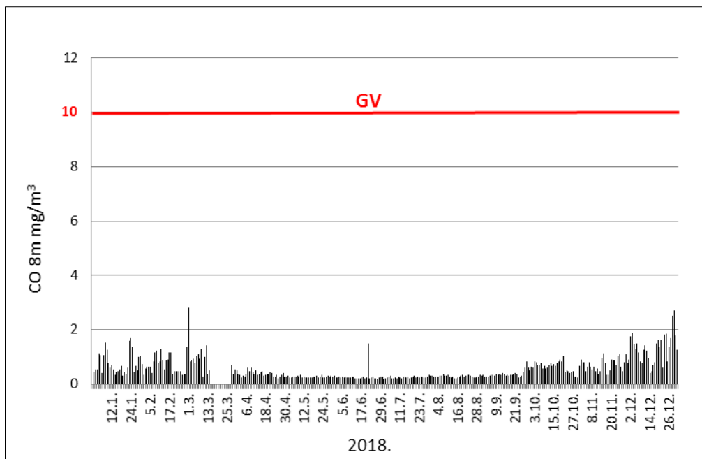
Slika 3.9. Kretanje srednjih 8-satnih koncentracija CO tijekom 2018. (Izrađeno prema podacima Ekonerga, 2019.)
