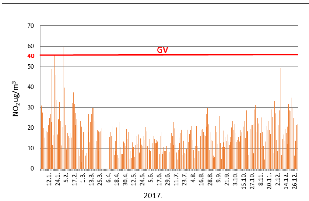
Slika 3.16. Kretanje srednjih 1-satnih koncentracija NO 2 tijekom 2017. (Izrađeno prema podacima Ekonerga, 2018.)
