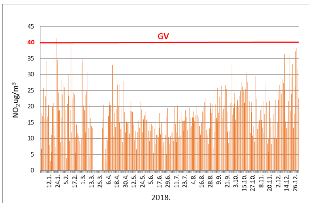
Slika 3.17. Kretanje srednjih 1-satnih koncentracija NO 2 tijekom 2018. (Izrađeno prema podacima Ekonega, 2019.)
